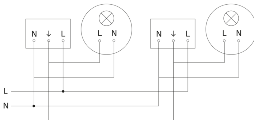
Diagrama electrónico interconexión varios sensores
