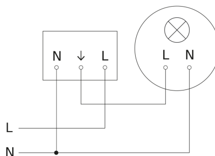
Diagrama electrónico
