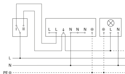
Diagrama electrónico conexión mediante un selector para funcionamiento de alumbrado permanente y automático
